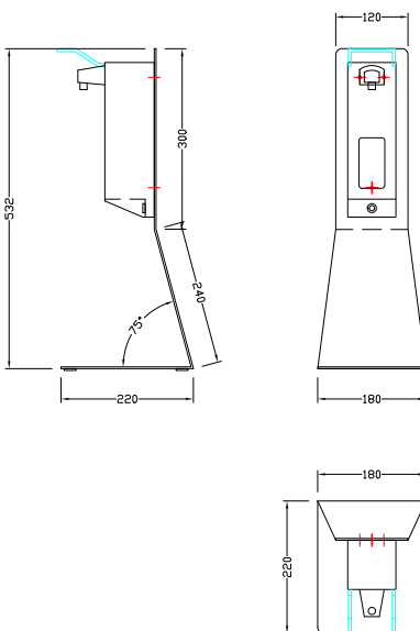
Art. Nr. TASAS Tisch Desinfektionsmittelständer aus Stahl 3 mm pulverbeschichtet RAL 9016 mit Aluminiumdispenser 0,5 Liter
