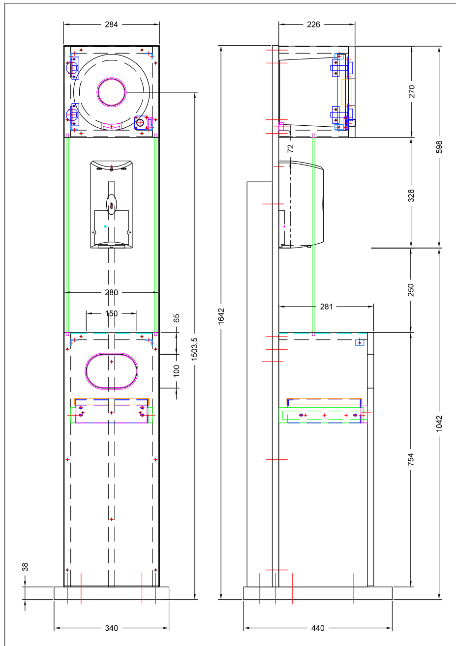
Abb.: Zeichnung mit Bemaßung (Hygienestation Variante 1)
