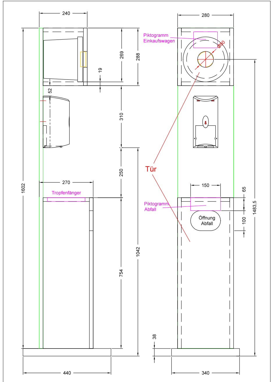
Abb.: Zeichnung mit Bemaßung (rote Variante)
