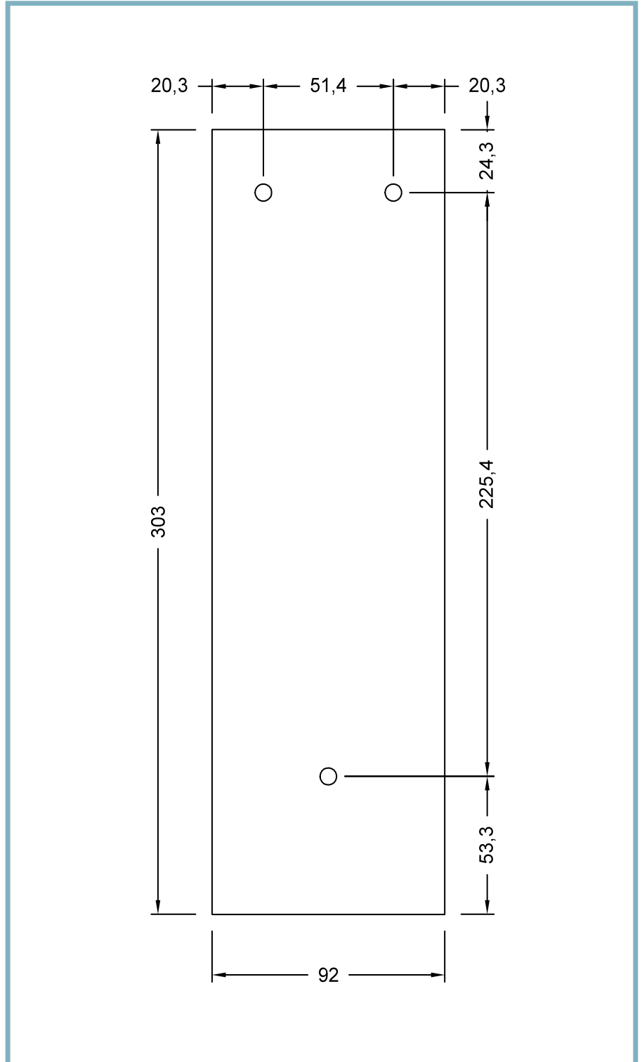
Zeichnung_01: Bohrmaße
