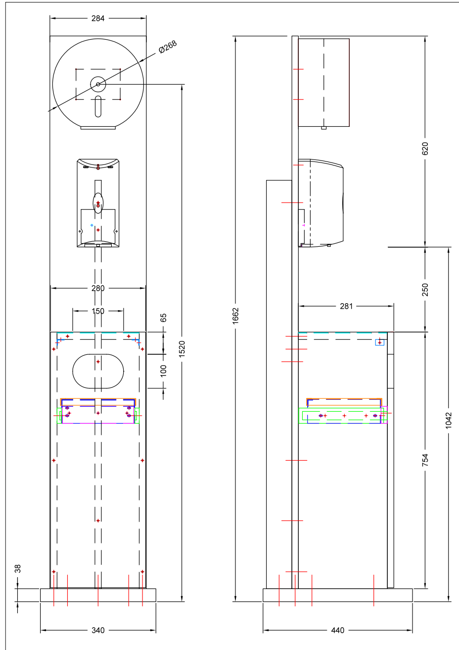
Abb.: Zeichnung mit Bemaßung (Hygienestation Variante 2)
